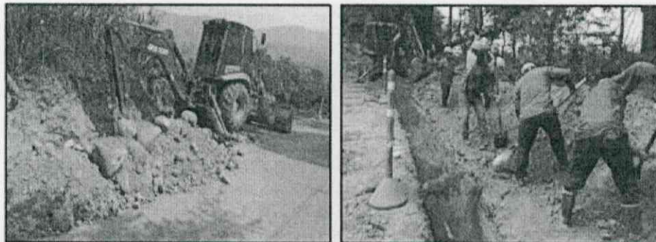
Imagen 15 Actividades relevantes del proyecto en ejecución "Construcción nueva línea de aducción de Ø14" PVC presión desde captación hasta la PTAP"
